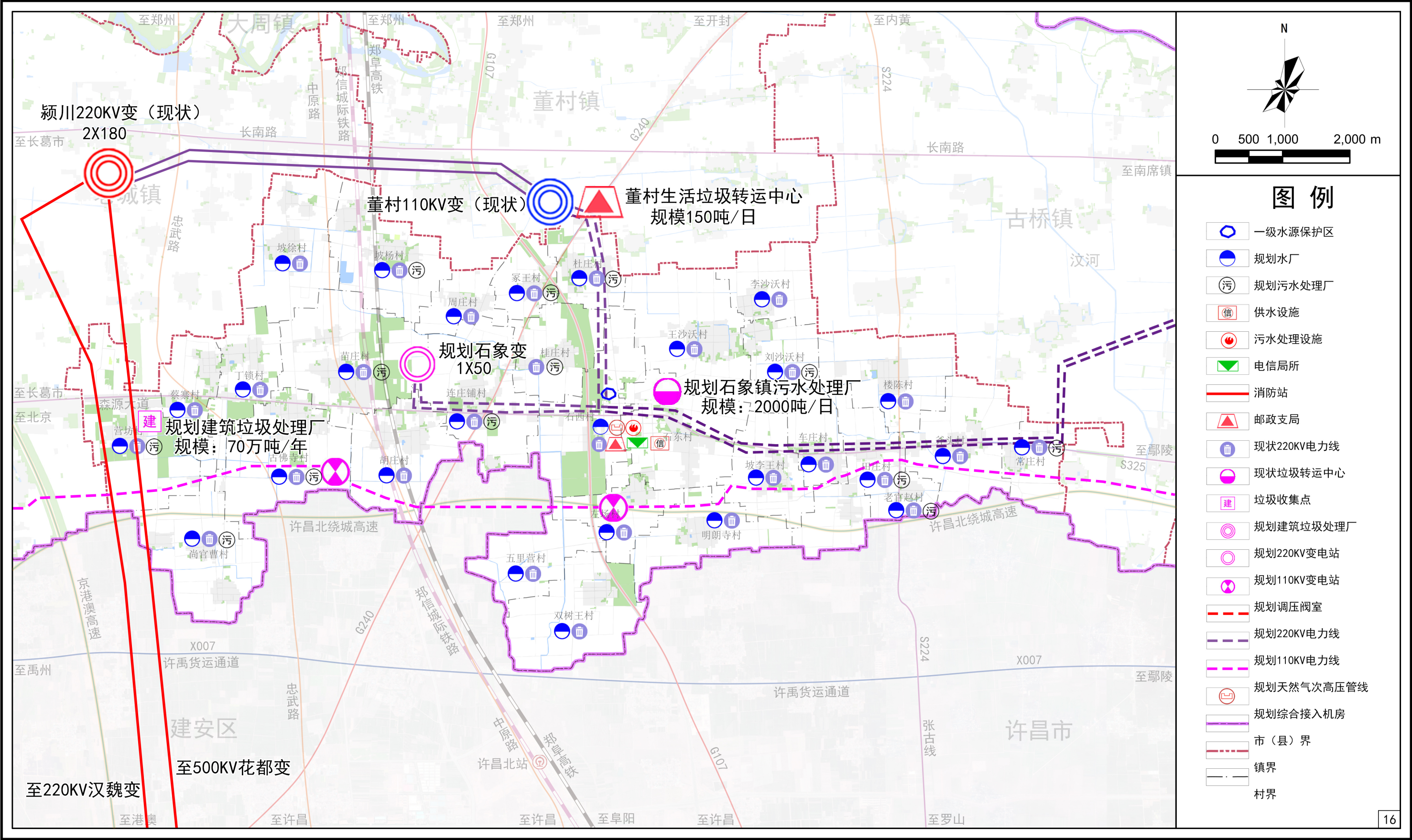
镇域基础设施规划图
